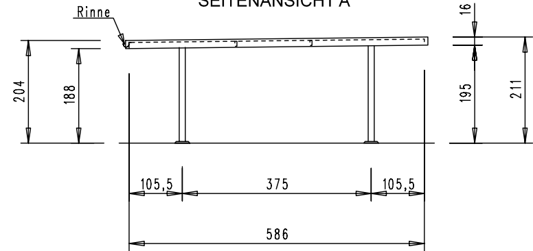
SEITENANSICHT A
